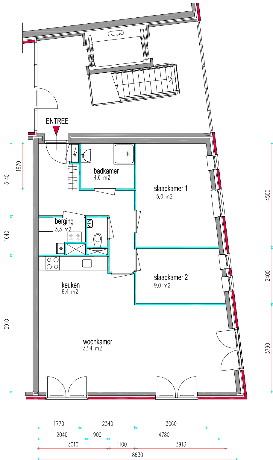
3e VERDIEPING
