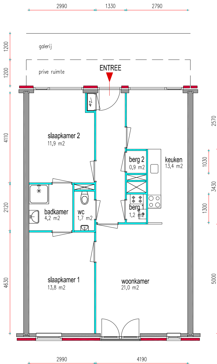
1e VERDIEPING
